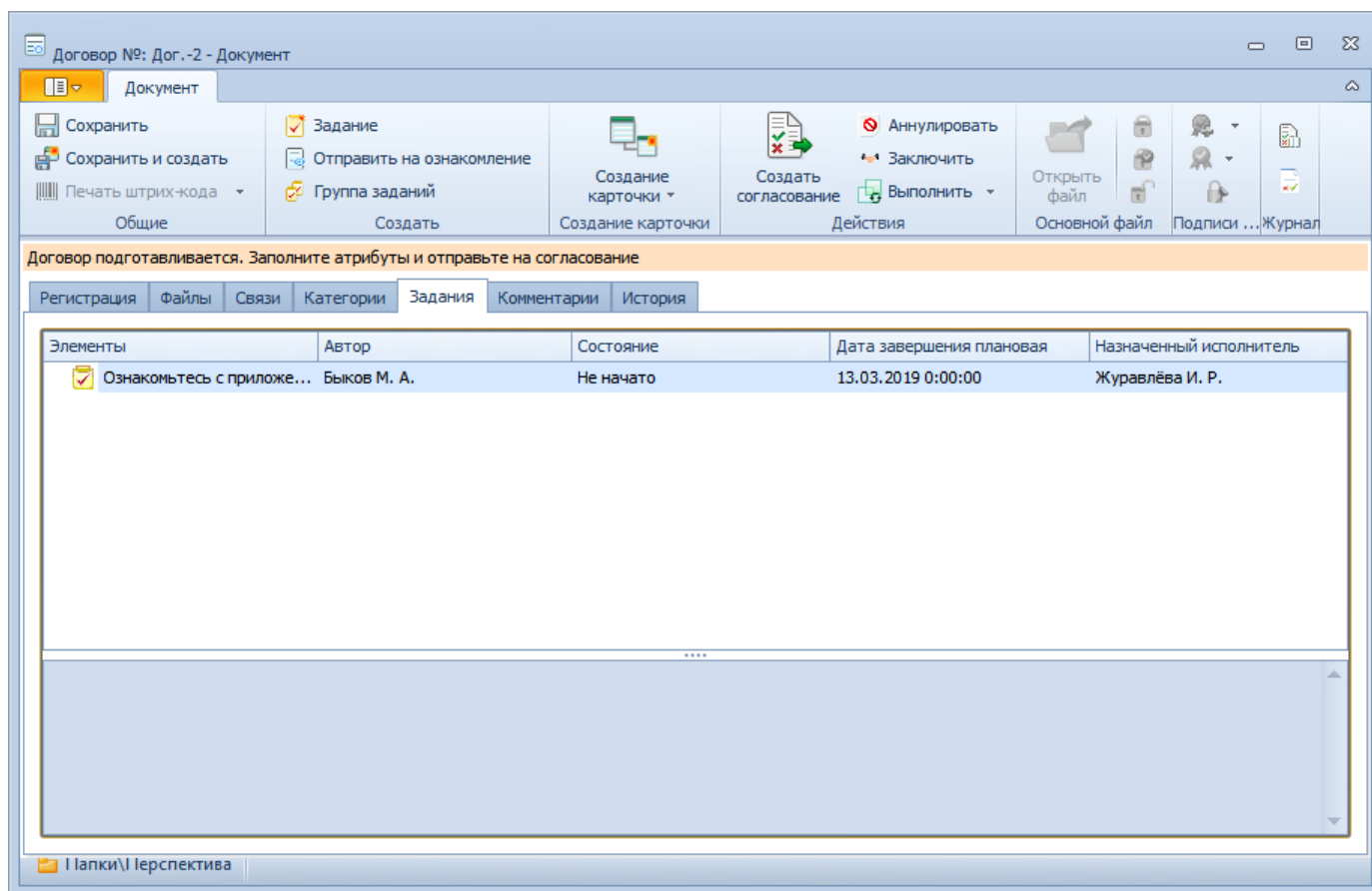
Рисунок 42. Вкладка "Задания"
