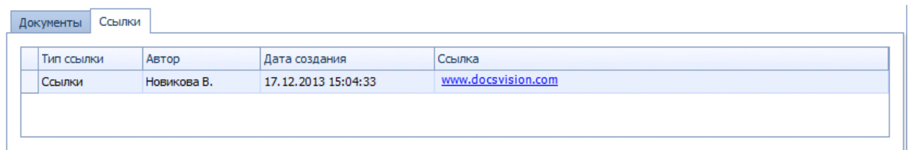
Рисунок 137. Добавление ссылок
