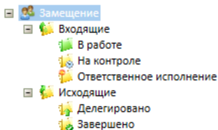
Рисунок 261. Папка "Замещение"
