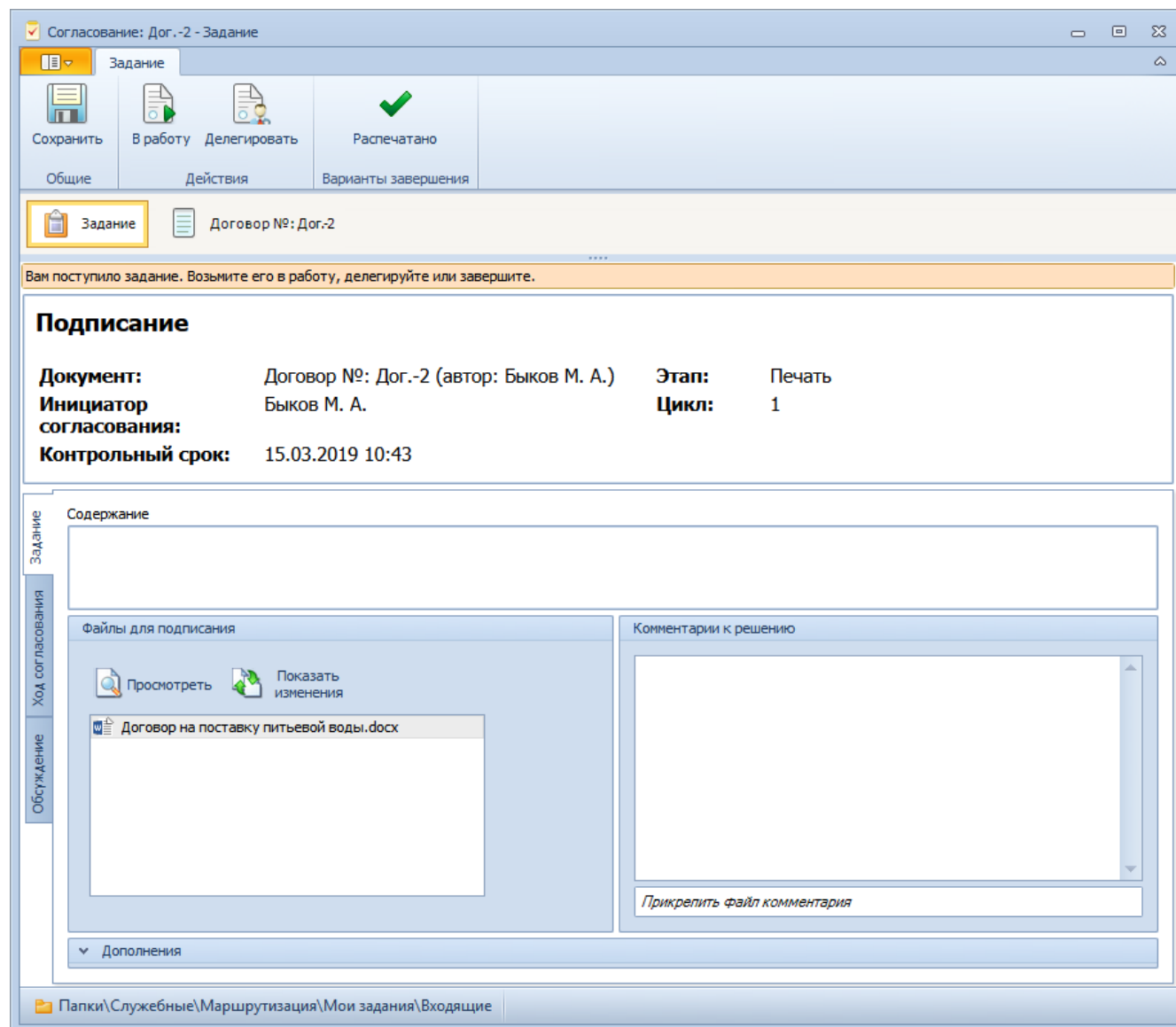
Рисунок 189. Печать договора
