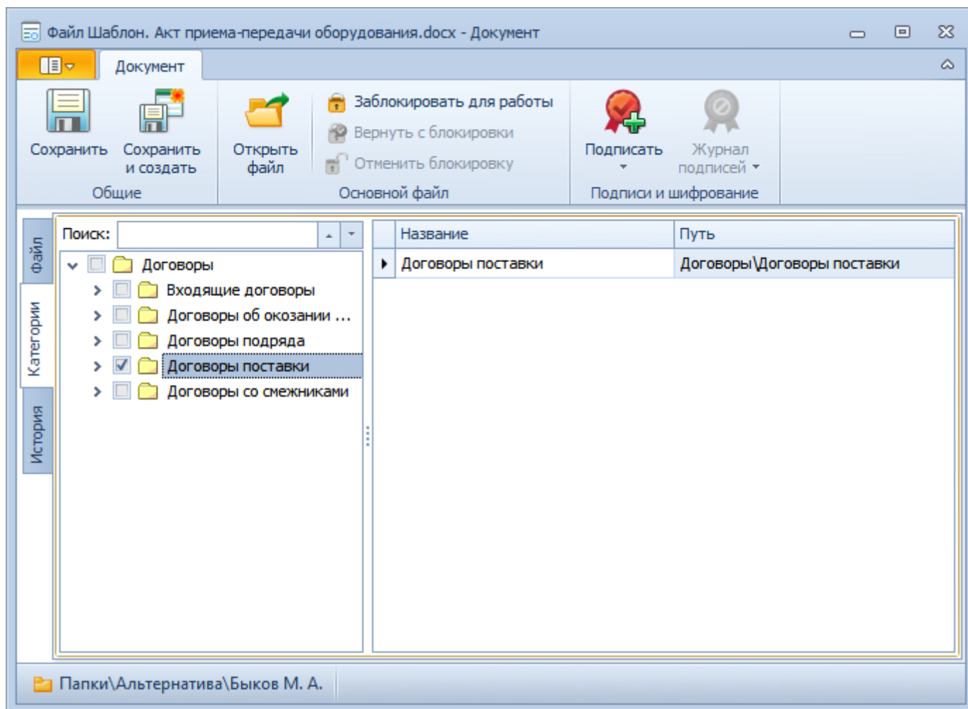
Рисунок 27. Вкладка "Категории"
