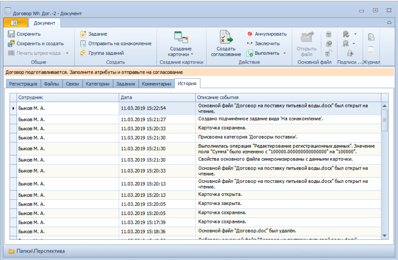
Рисунок 44. Вкладка "История"
