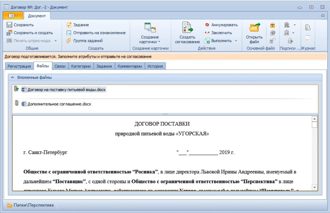
Рисунок 39. Вкладка "Файлы"
