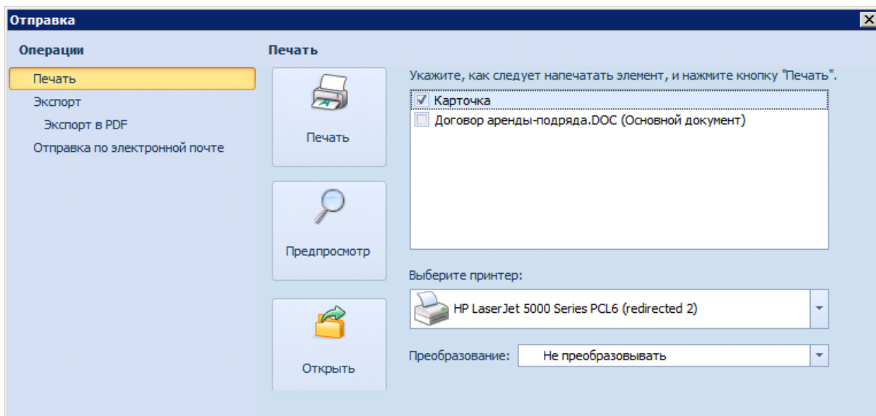
Рисунок 99. Печать карточки
