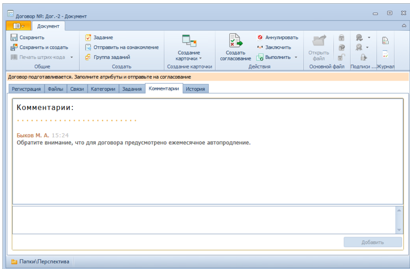
Рисунок 43. Вкладка "Комментарии"
