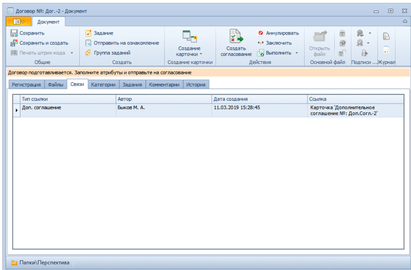
Рисунок 40. Вкладка "Связи"
