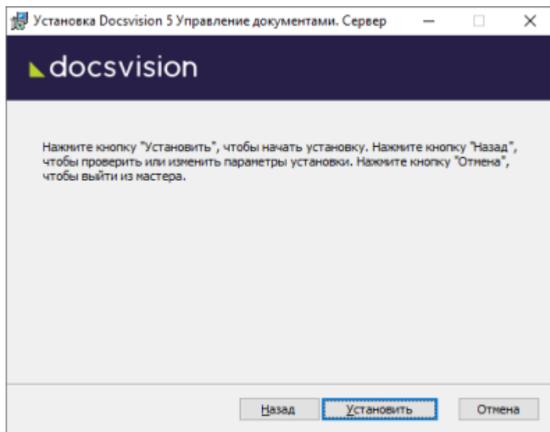
Рисунок 220. Подтверждение установки
