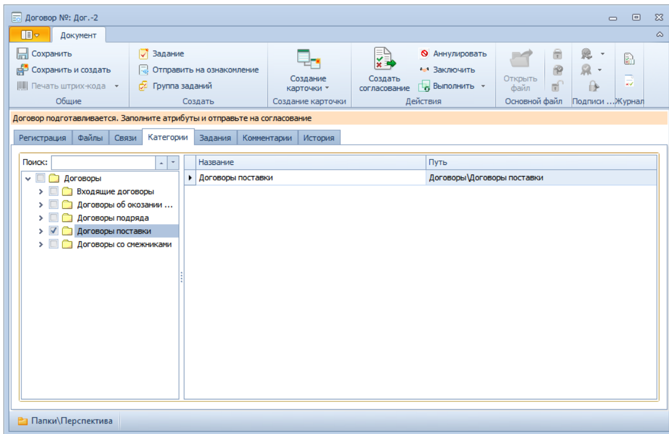
Рисунок 41. Вкладка "Категории"
