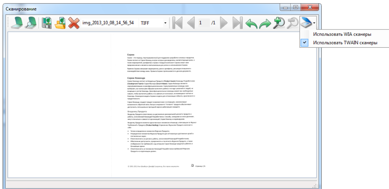
Рисунок 93. Окно "Сканирование"
