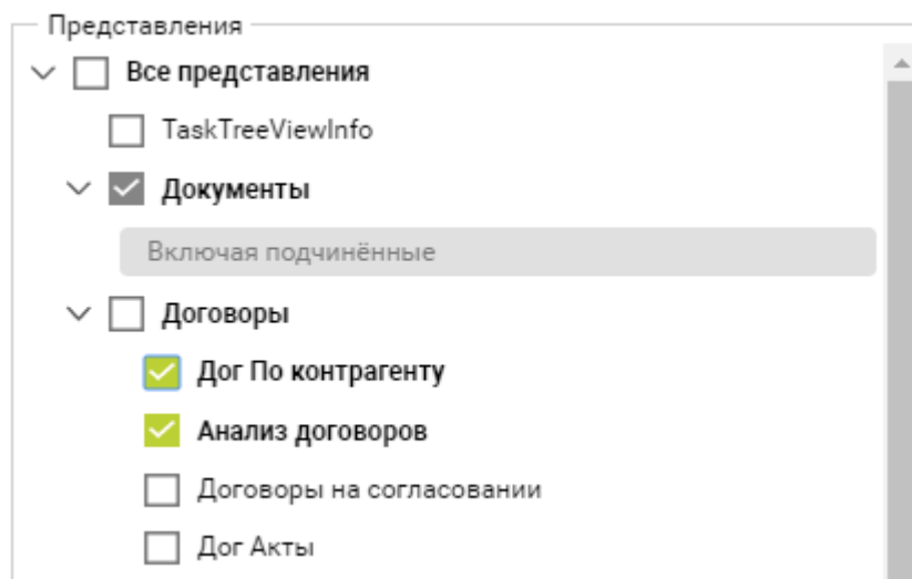
Рисунок 37. Дерево представлений с выбранными представлениями
