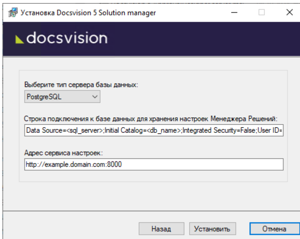
Рисунок 5. Подключение к базе данных Менеджера решений
