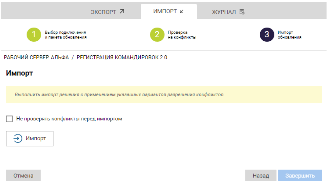
Рисунок 55. Страница "Импорт обновления"
