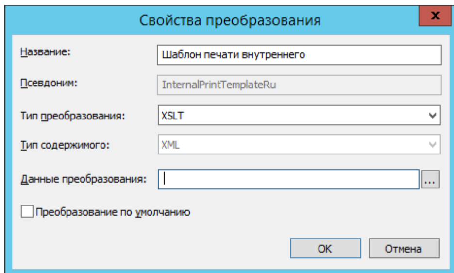
Рисунок 161. Свойства преобразования карточки
