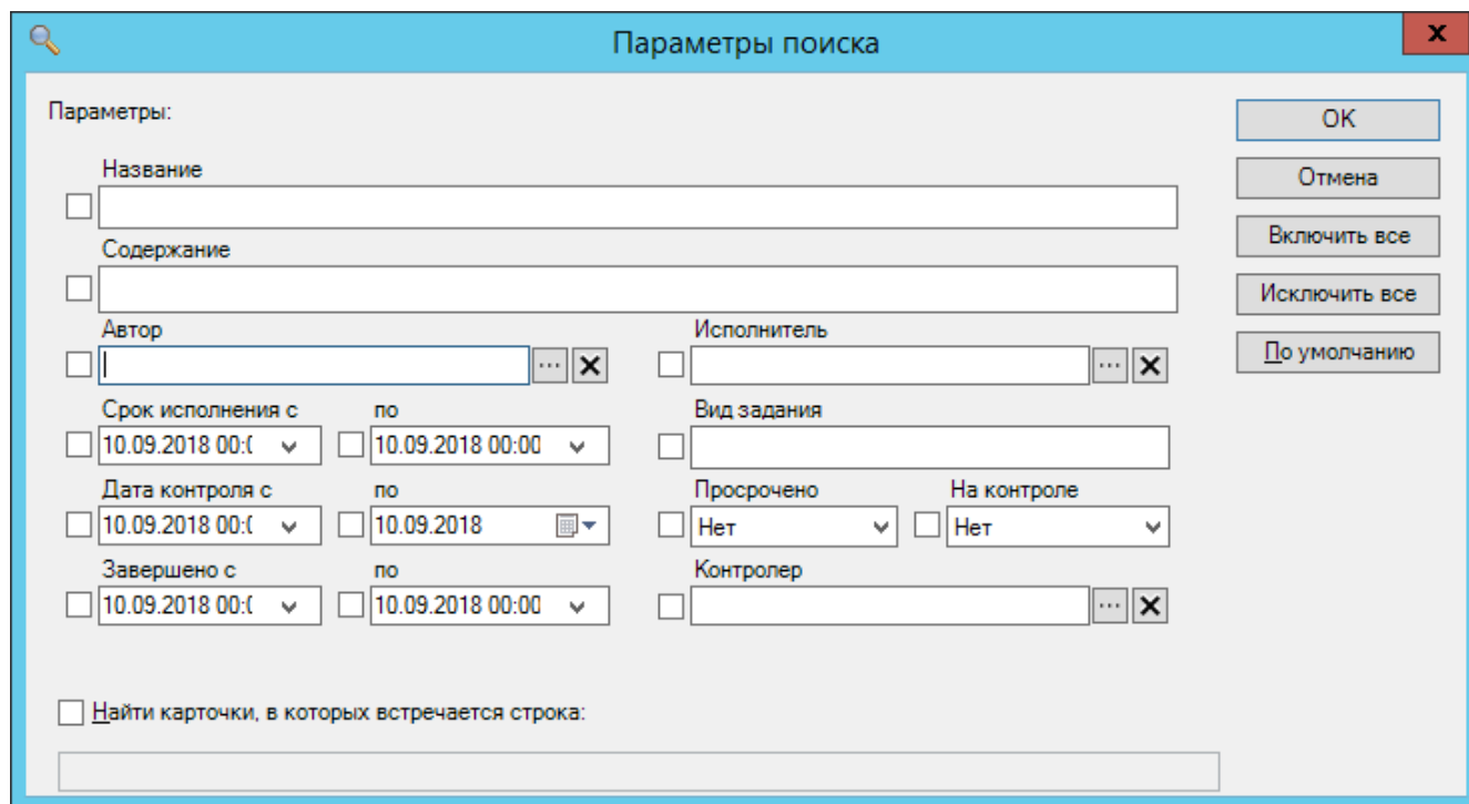
Рисунок 106. Пример окна для настройки параметров атрибутивного поиска
