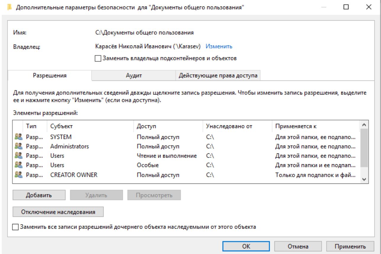
Рисунок 59. Вкладка "Безопасность" окна свойств стандартной папки
