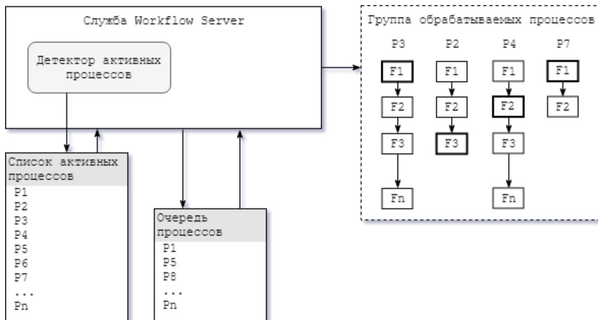
Рисунок 2. Схема работы службы "Workflow Server"
