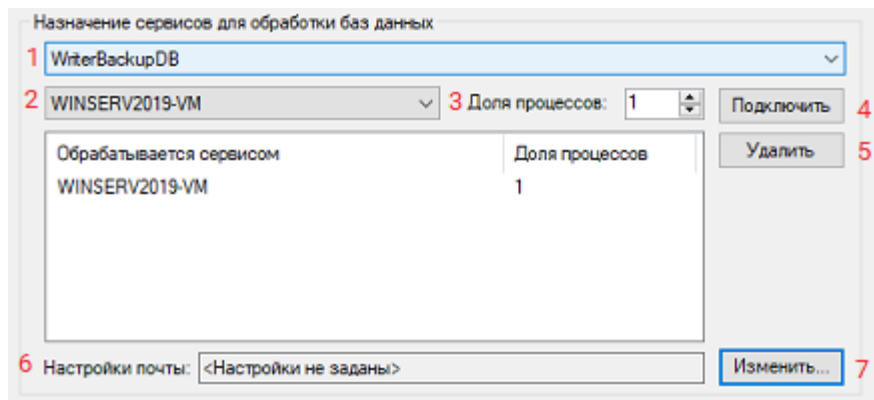
Рисунок 17. Блок "Назначение сервисов для обработки баз данных"
