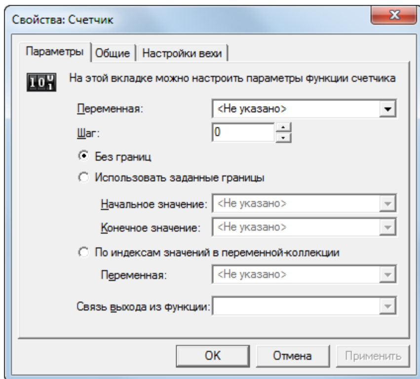
Рисунок 72. Окно "Счетчик". Вкладка "Параметры"
