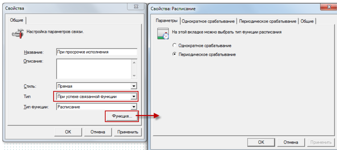
Рисунок 57. Окно параметров связи и связанной функции
