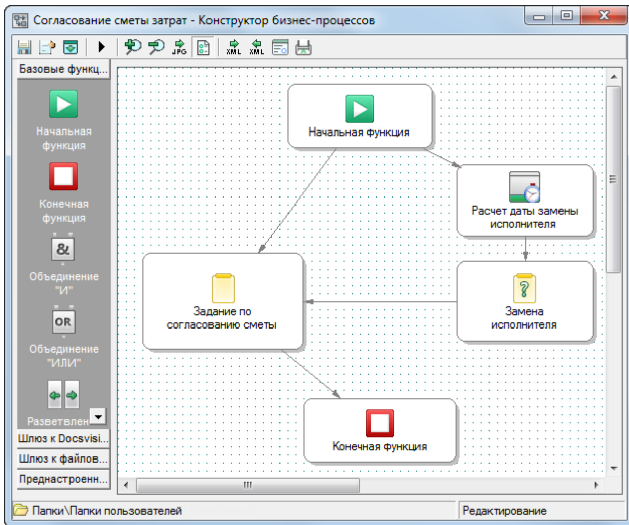
Рисунок 132. Пример работы функции управления заданием
