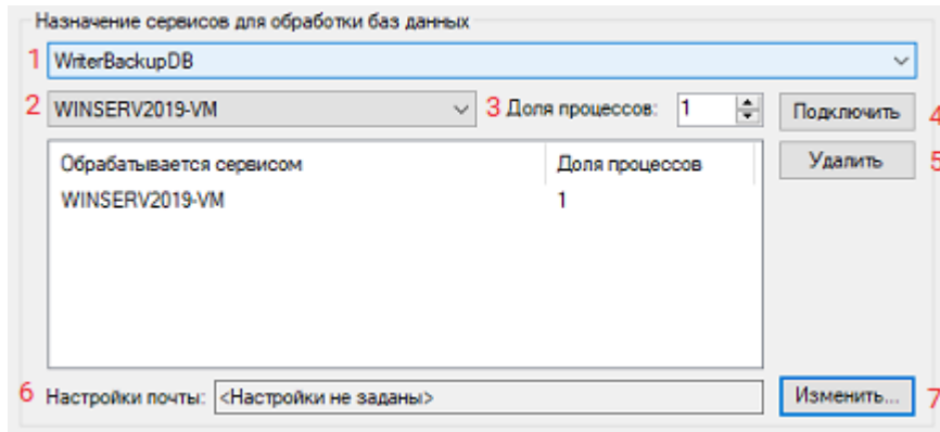
Рисунок 14. Блок "Назначение сервисов для обработки баз данных"
