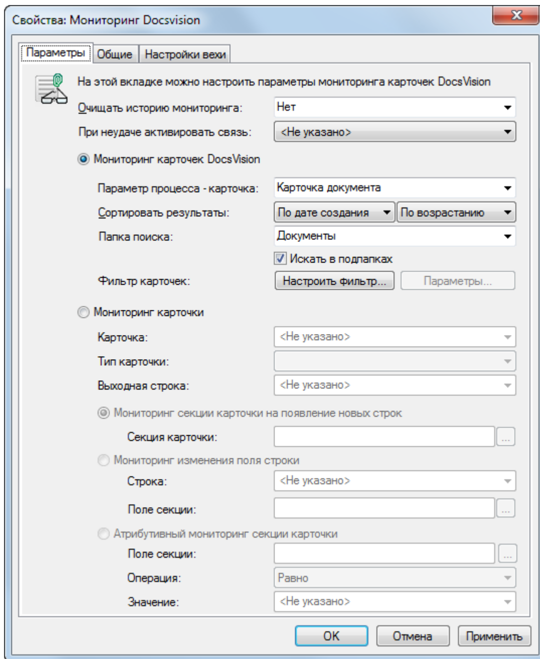
Рисунок 96. Свойства функции "Мониторинг Docsvision". Вкладка "Параметры"
