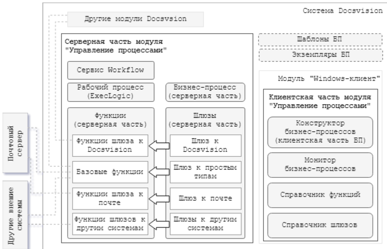
Рисунок 1. Архитектура модуля Управление процессами
