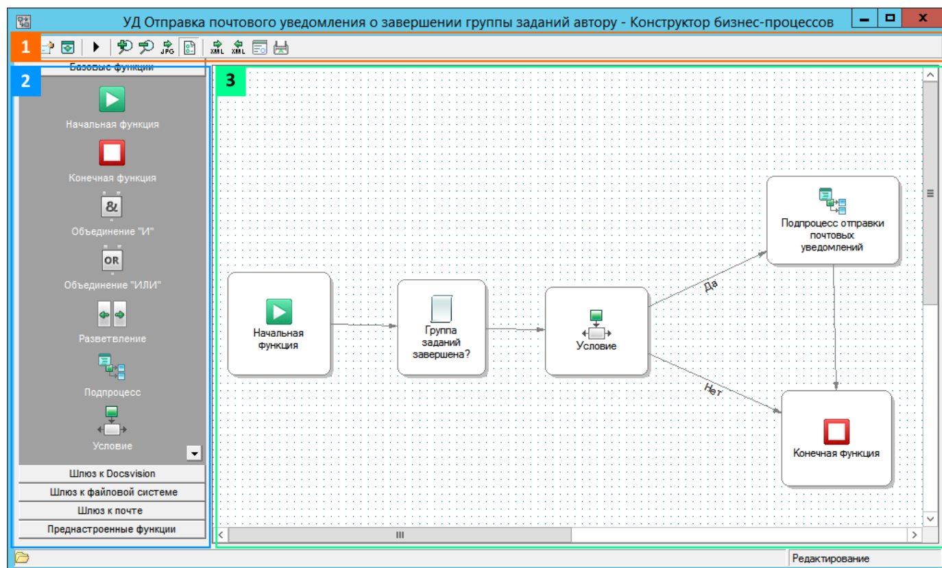
Рисунок 40. Обычный режим работы "Конструктора бизнес-процессов"
