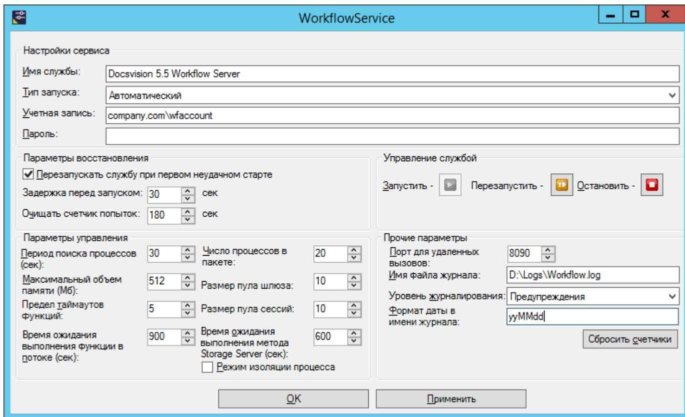
Рисунок 16. Окно настройки сервиса Workflow
