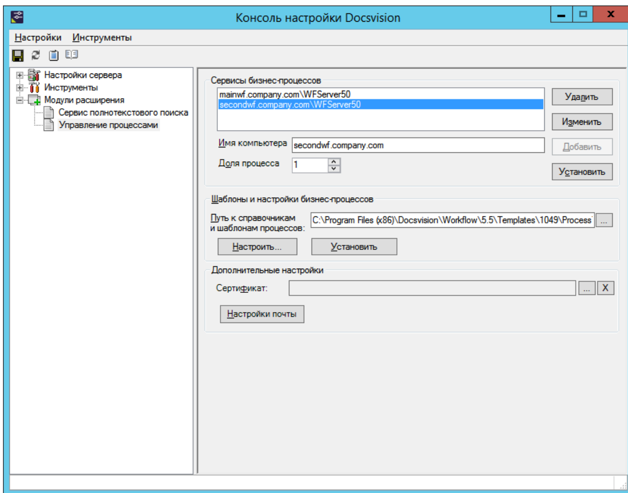
Рисунок 34. Настройки кластеризации модуля Управление процессами
