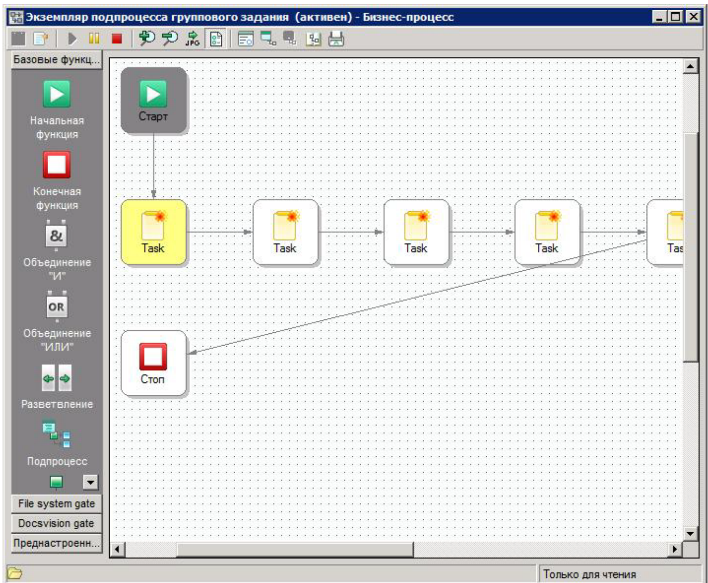
Рисунок 116. Экземпляр подпроцесса группового задания для функции "Последовательное задание"
