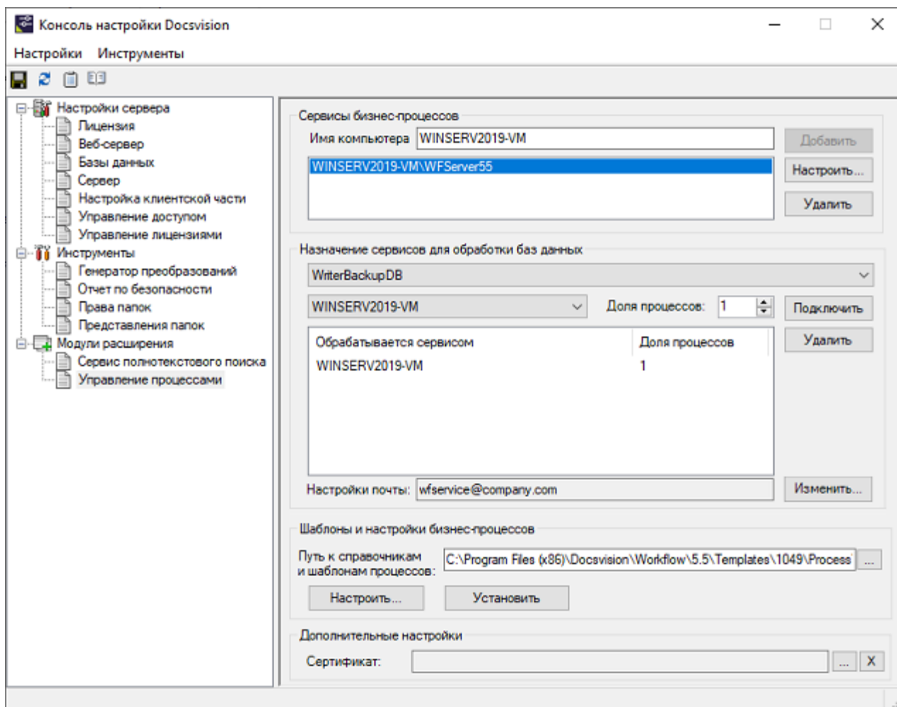
Рисунок 13. Раздел настроек Управление процессами консоли настройки Docsvision
