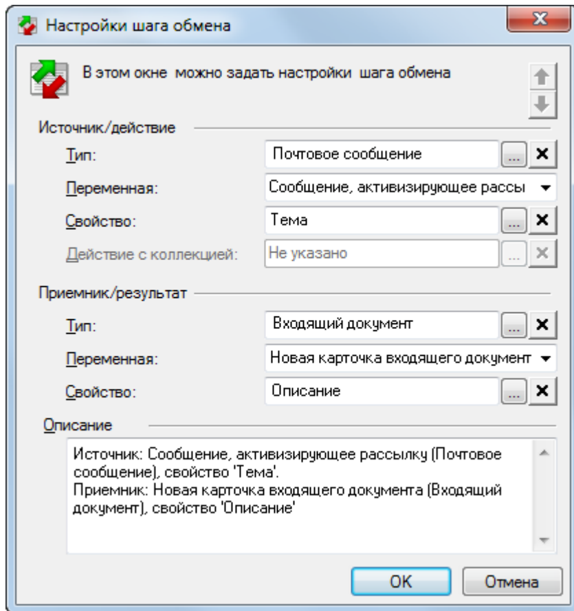
Рисунок 88. Окно "Настройки шага обмена"
