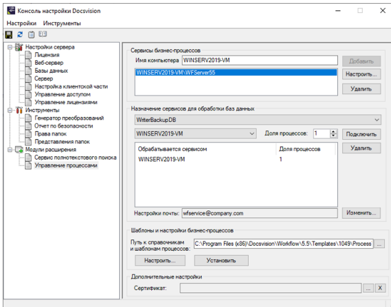
Рисунок 10. Раздел настроек Управление процессами консоли настройки Docsvision
