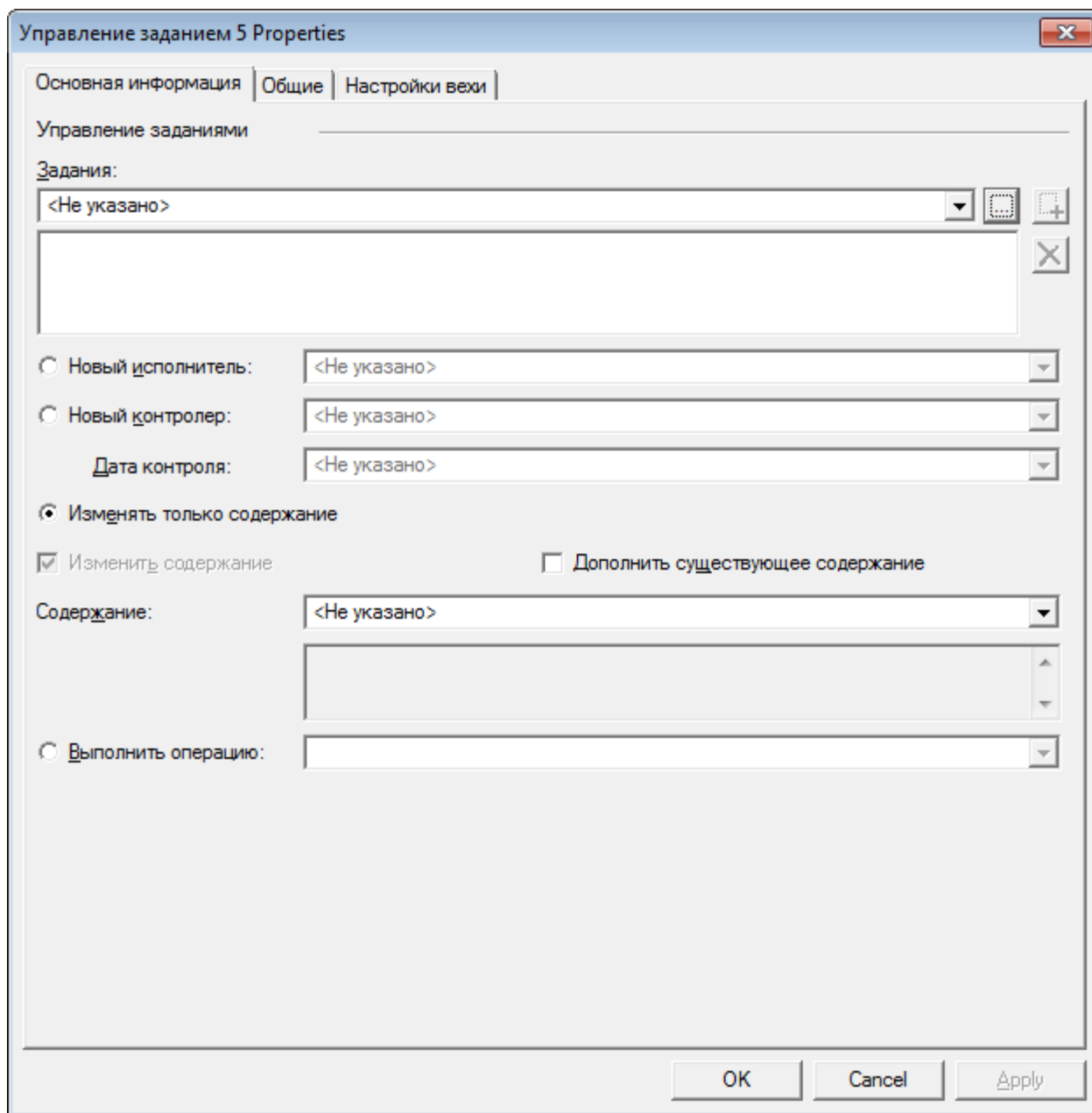
Рисунок 110. Свойства функции "Управление заданием 5". Вкладка "Основная информация"
