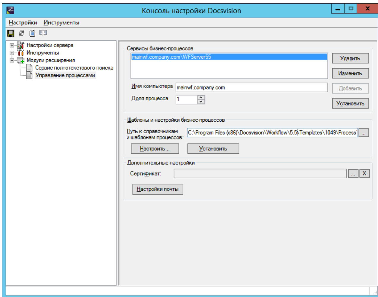
Рисунок 33. Базовые настройки модуля Управление процессами
