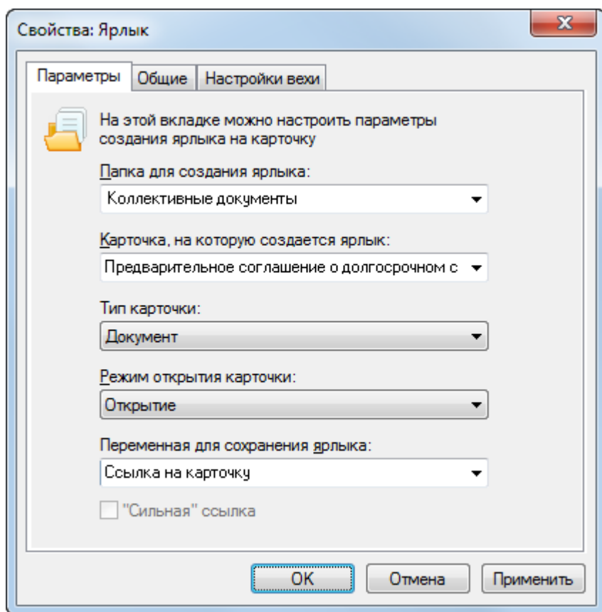
Рисунок 99. Свойства функции "Ярлык". Вкладка "Параметры"
