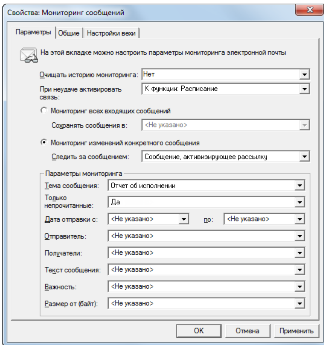
Рисунок 143. Свойства функции "Мониторинг сообщений". Вкладка "Параметры"
