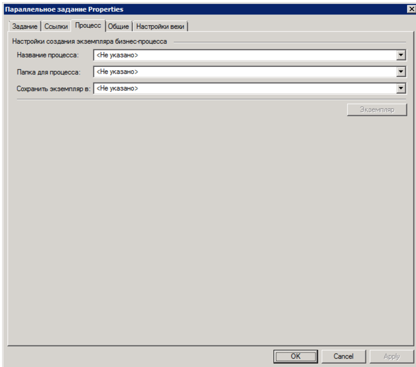
Рисунок 114. Свойства функции "Параллельное задание". Вкладка "Процесс"
