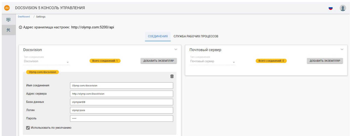
Рисунок 8. Адрес сервиса настроек также отображается на странице соединений
