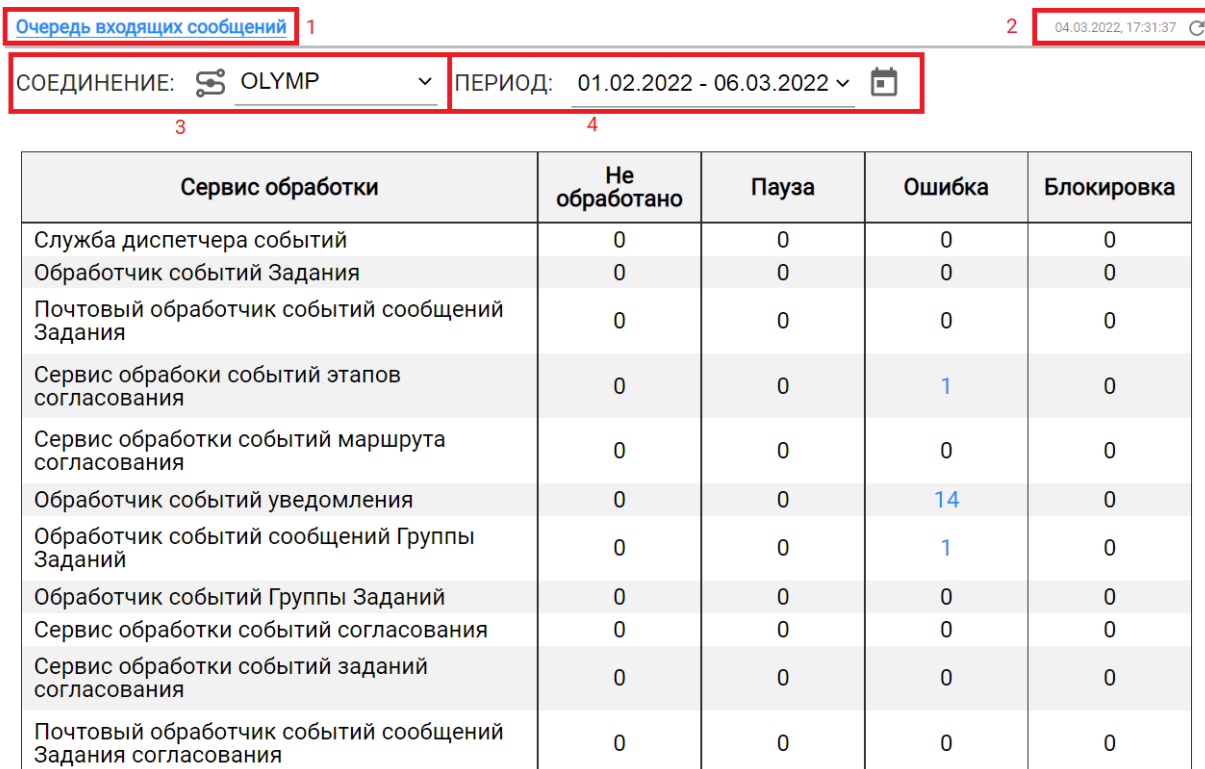
Рисунок 32. Текстовый виджет "Очередь входящих сообщений"
