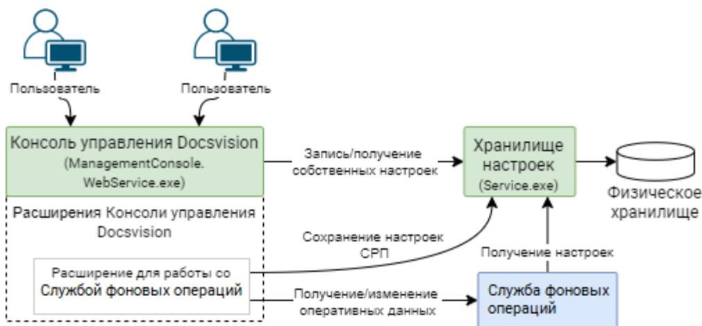
Рисунок 1. Схема работы Консоли управления Docsvision
