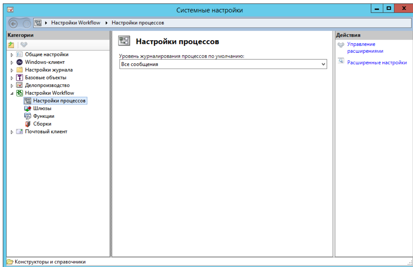
Рисунок 20. Настройки процессов
