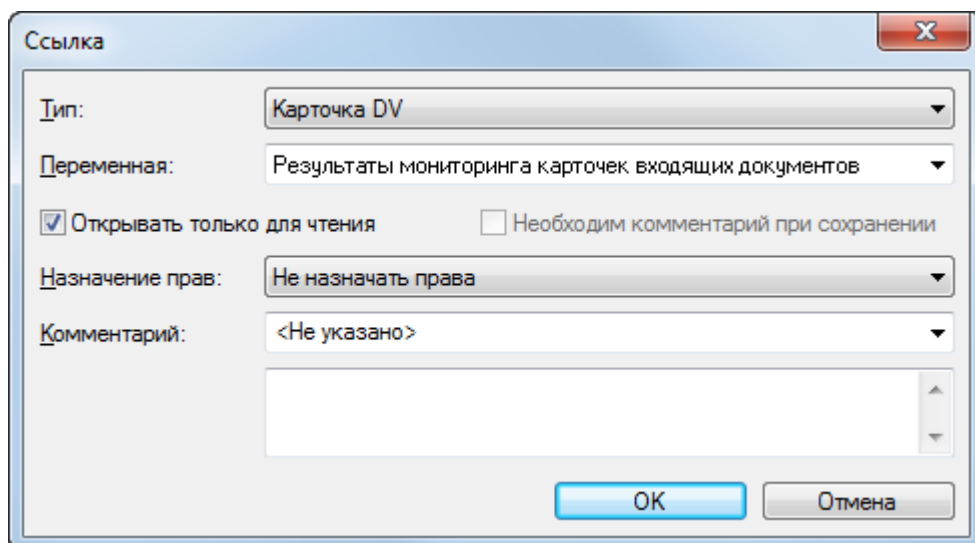
Рисунок 114. Окно "Ссылка"
