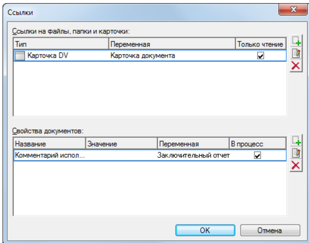
Рисунок 113. Окно "Ссылки"
