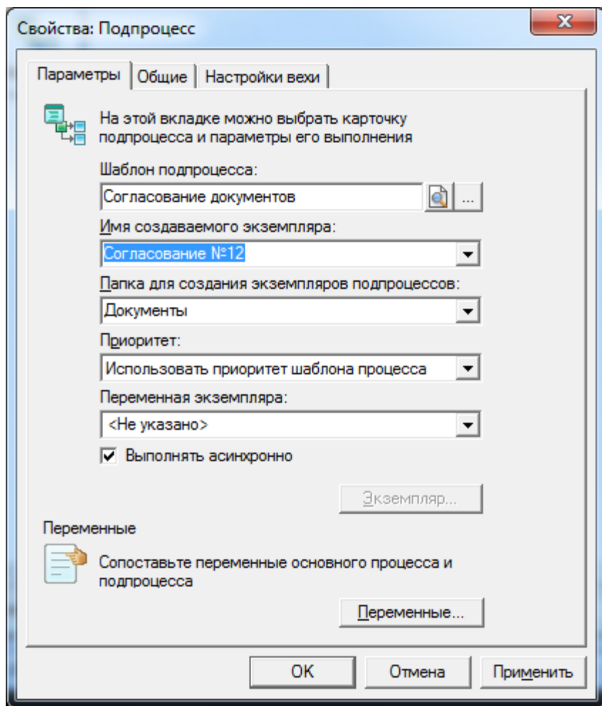
Рисунок 55. Параметры подпроцесса
