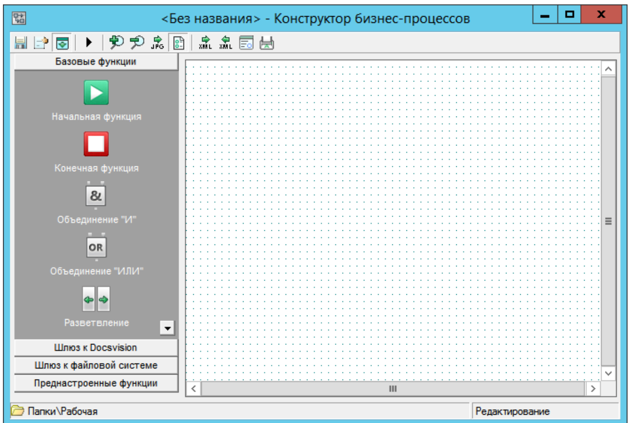
Рисунок 34. Конструктор бизнес-процессов
