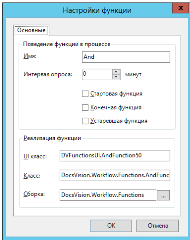
Рисунок 24. Настройки функции
