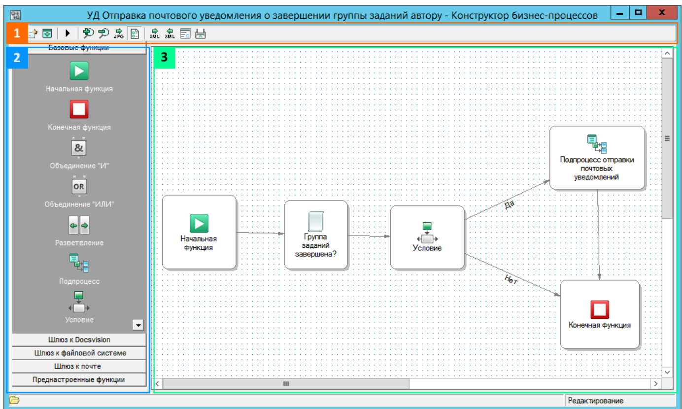
Рисунок 2. Конструктор бизнес-процессов
