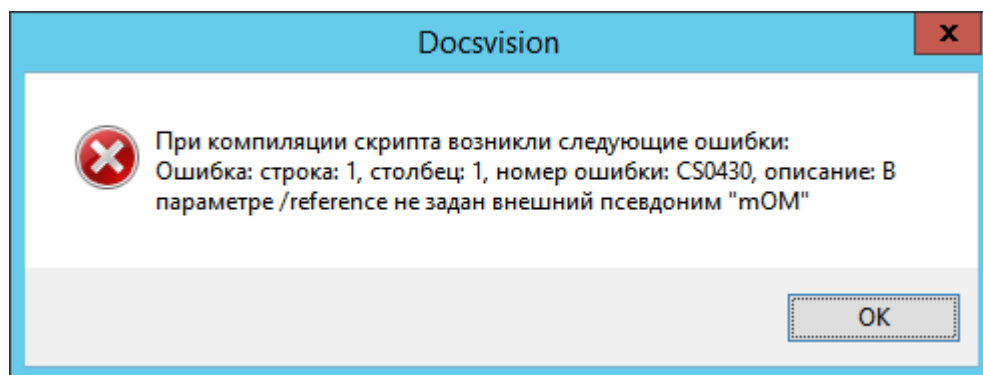
Рисунок 48. Окно ошибки
